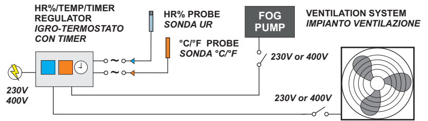
EC100021 Schema esemplificativo installazione - Mounting layout example
